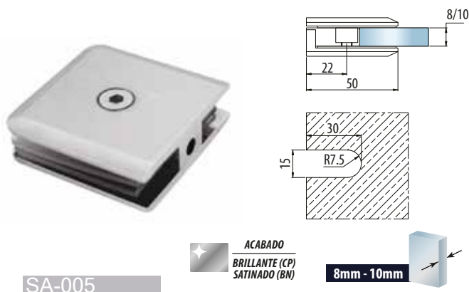
Conector vidrio - muro
