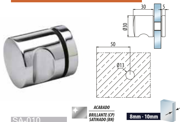
Botón de ducha sencillo
