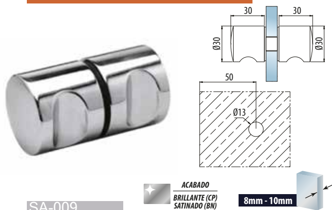
Botón de ducha doble
